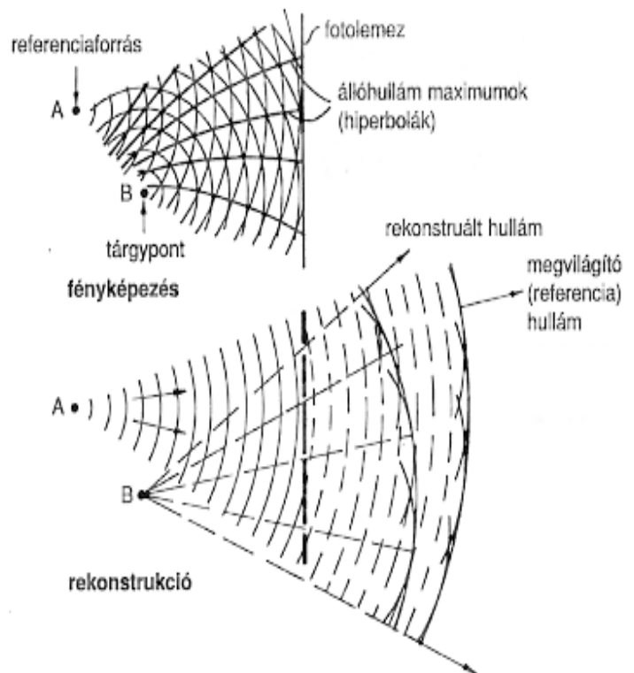
2. ábra. A holográfia alapelve, 1947.
